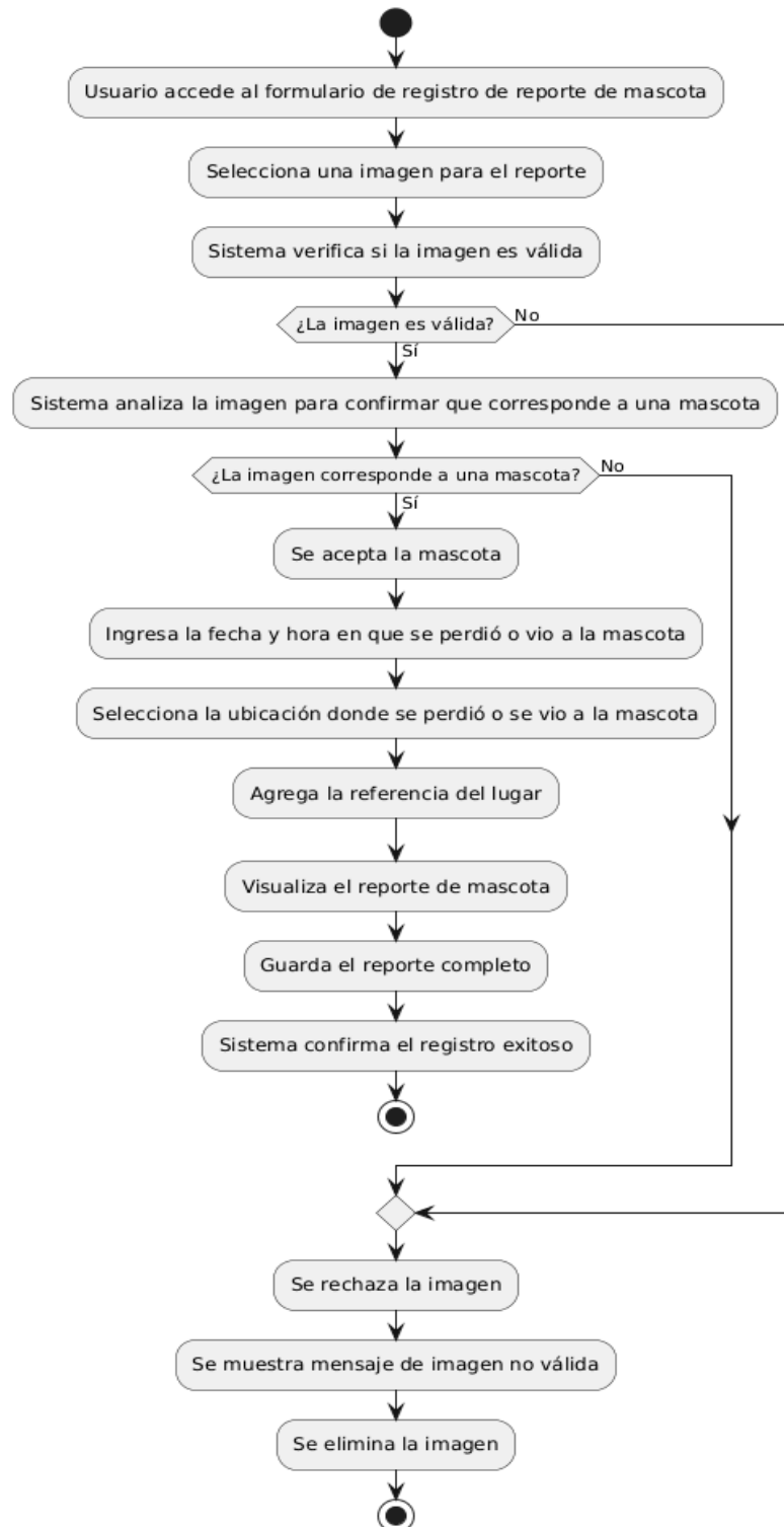
Figura 10: Diagrama de Actividades con Objetos de Registrar reporte de mascota fase análisis
