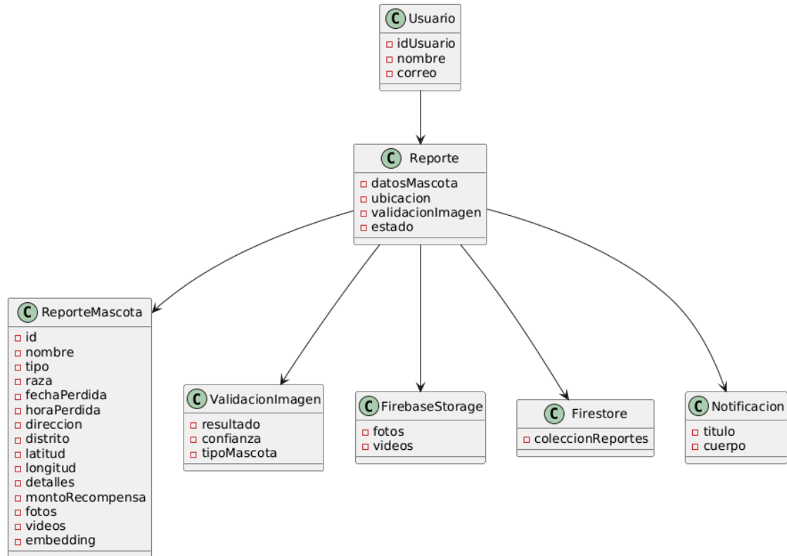
Figura 39: Diagrama de Caso de Clases de Registrar reporte de mascota fase análisis
