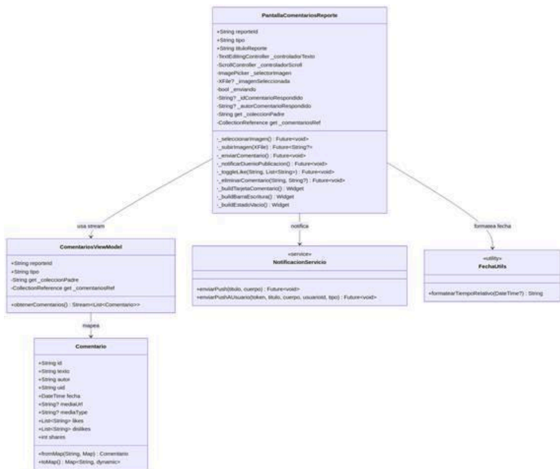
Figuras 04 (análisis) y 09 (diseño). Diagrama de clases de Gestionar Comentarios.
